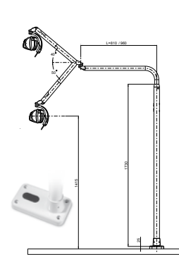
BODENADAPTION
